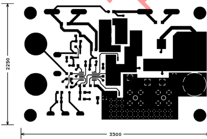
Top Layer
