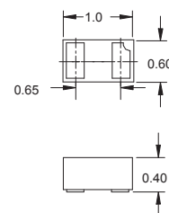
SLP1006P2T
